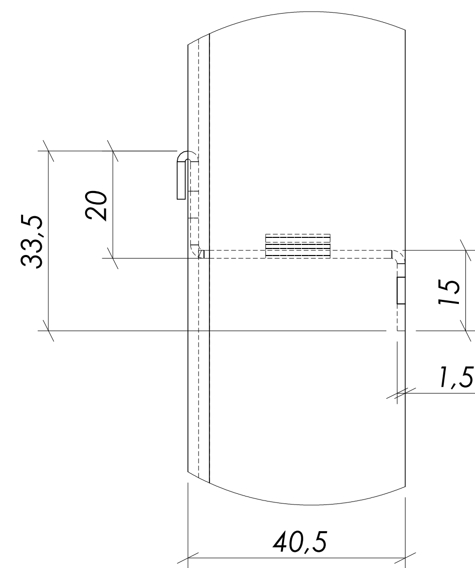
SZCZEGÓŁ B
