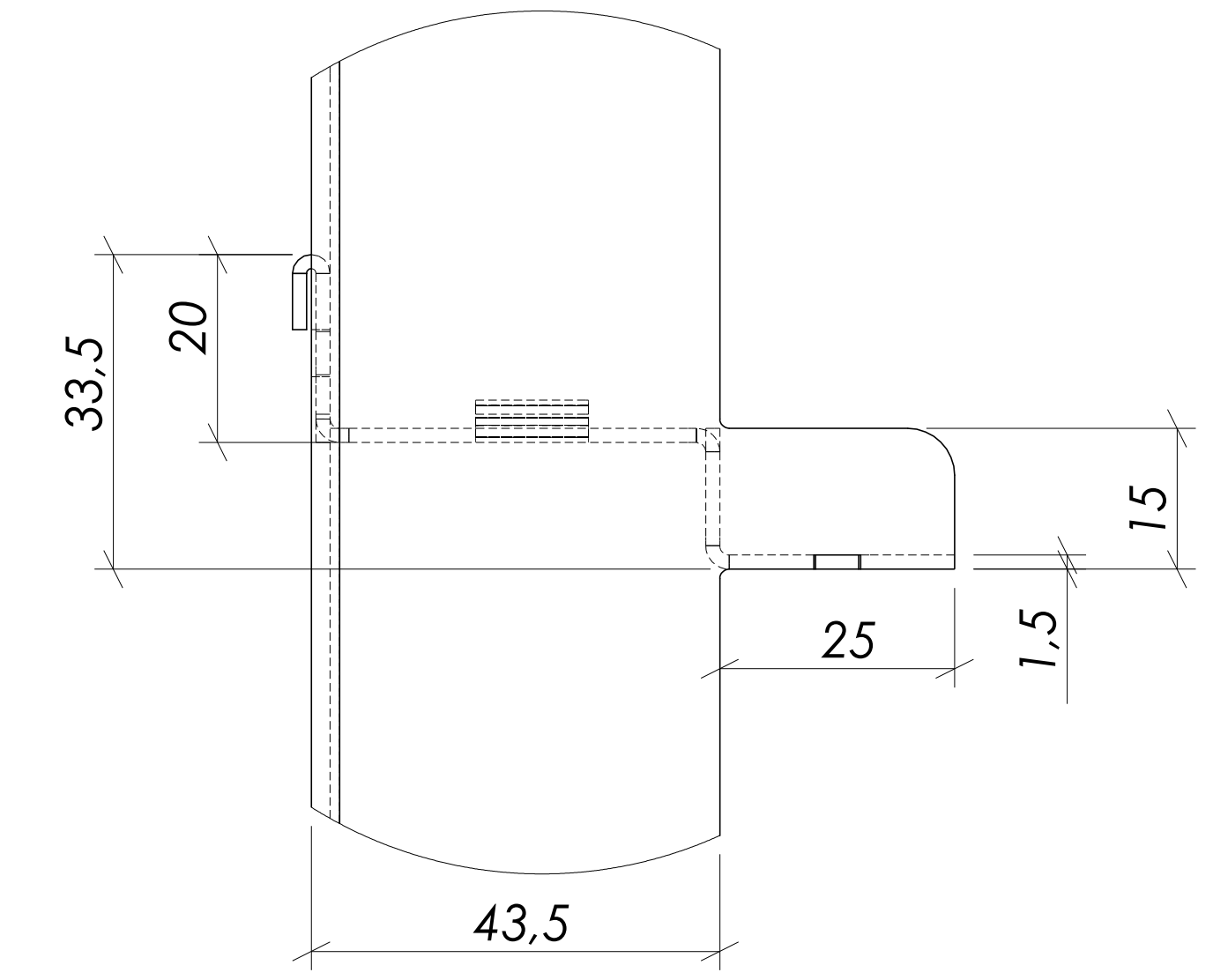
SZCZEGÓŁ B
