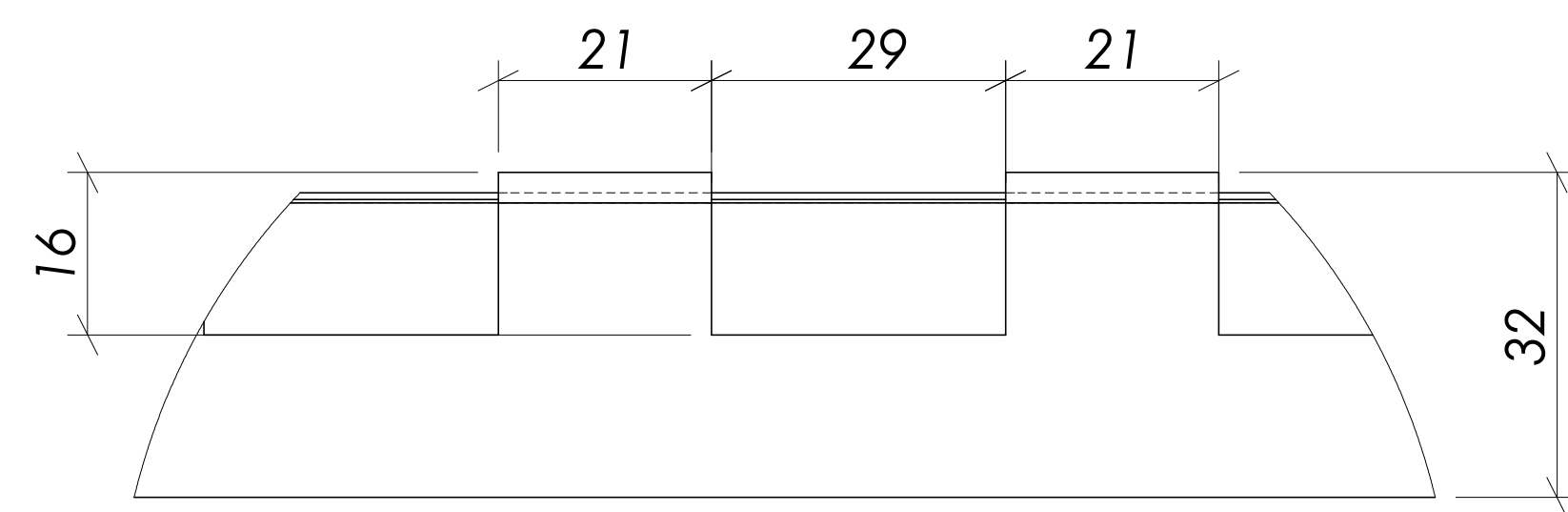
SZCZEGÓŁ C
