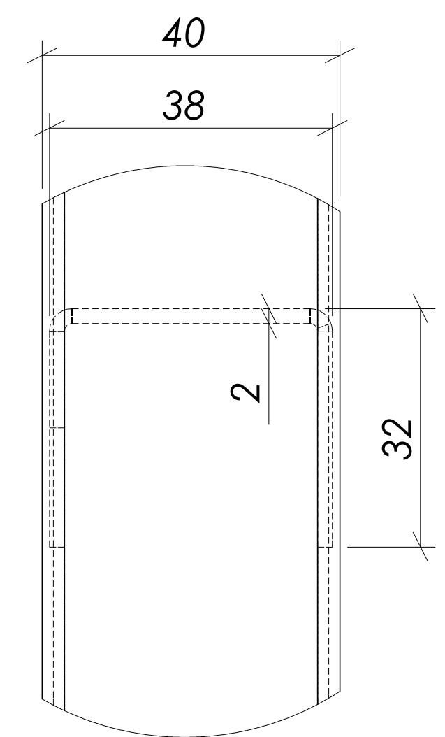
SZCZEGÓŁ A
